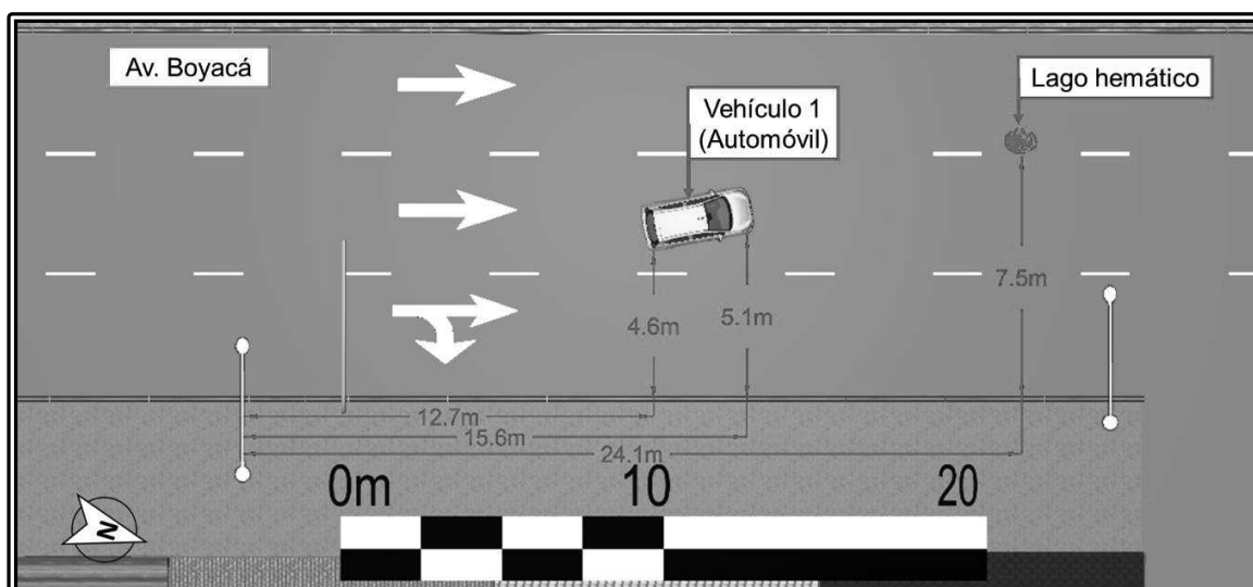
Imagen 2.10 Plano de la escena
