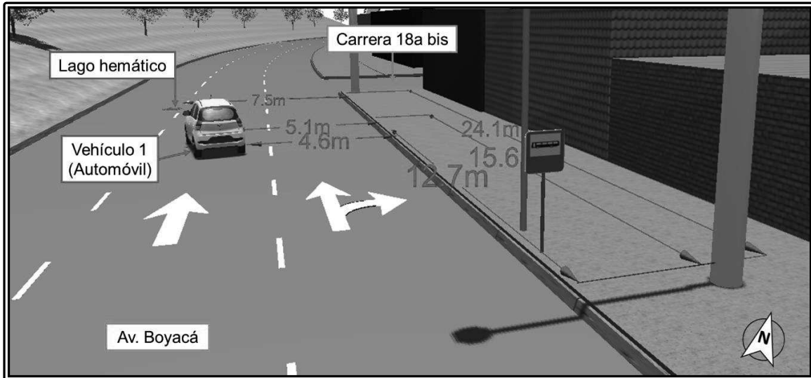
Imagen 2.11 Plano de la escena
