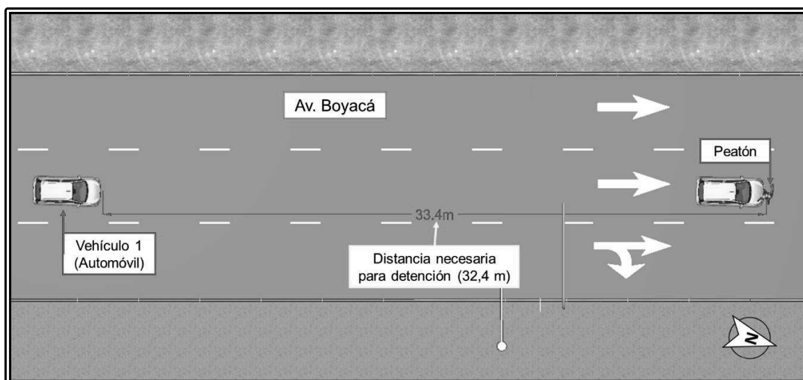
Imagen 4.11 Zona de percepción reacción
