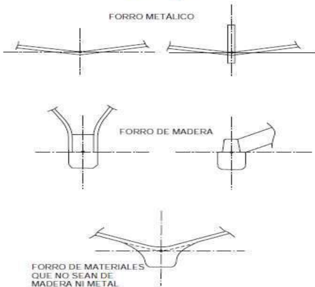
Figura 3 Línea de quilla
