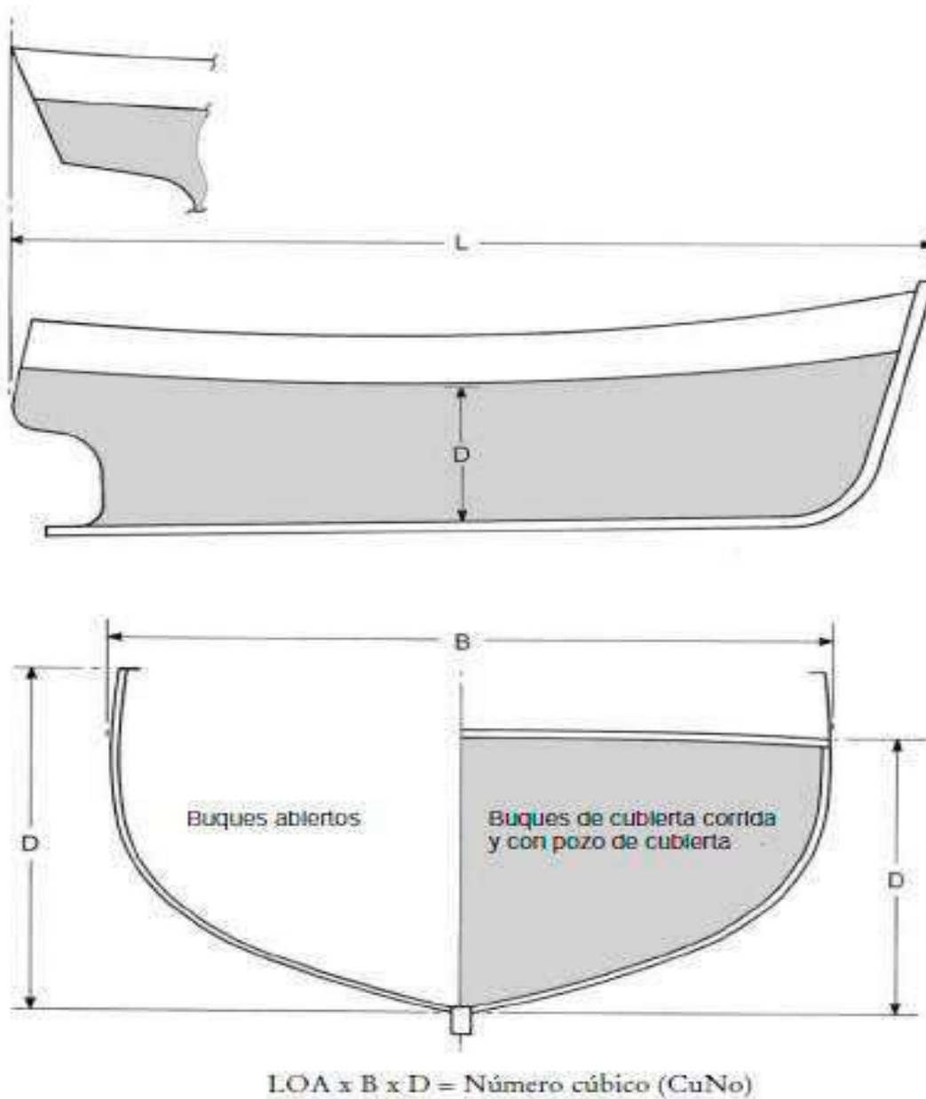
Figura 6 Número cúbico
