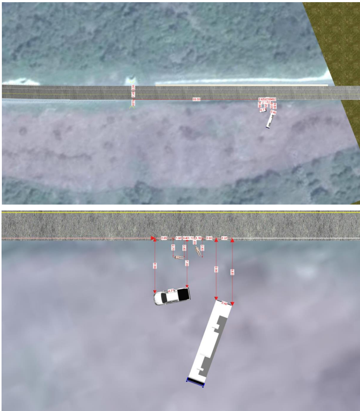
IMAGEN No. 19: En estas imágenes, vista en planta se aprecian las evidencias diagramadas en el croquis del informe de la autoridad y el ajuste realizado con base a las fichas técnicas de los vehículos y fotografías del día de los hechos.
