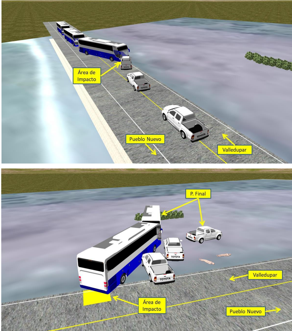
IMAGEN No. 26: En estas imágenes en 3D se aprecia la secuencia del accidente, nótese el sentido de desplazamiento de los vehículos y la posición relativa al momento del impacto y los desplazamientos hasta sus posiciones finales.
