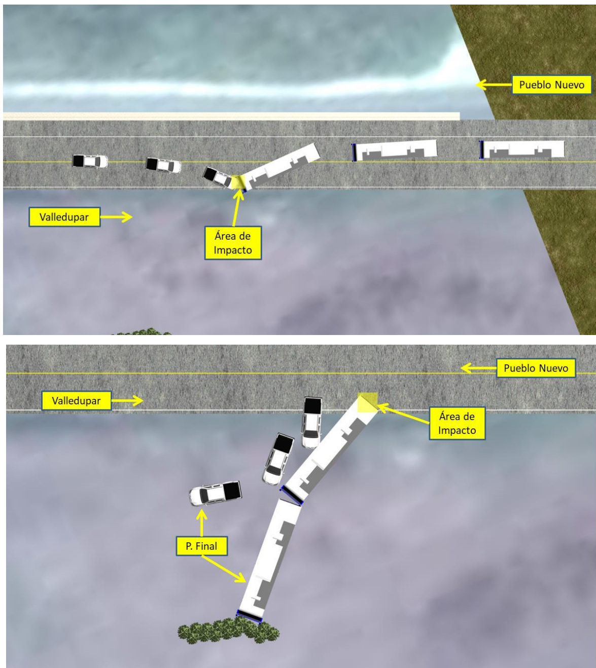
IMAGEN No. 25: En estas imágenes, vista en planta, se aprecia la secuencia del siniestro, nótese el sentido de desplazamiento de los vehículos, el área de impacto de color amarillo y el movimiento hasta sus posiciones finales.
