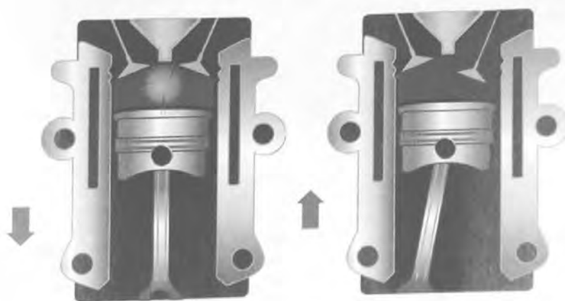
El motor Otto (tradicional) y el Atkinson tienen idéntico funcionamiento en las fases de admisión, combustión y escape, típicas de la maquinaria de cuatro tiempos.
