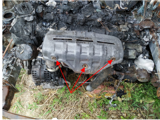
Aislante térmico sin tornillería
