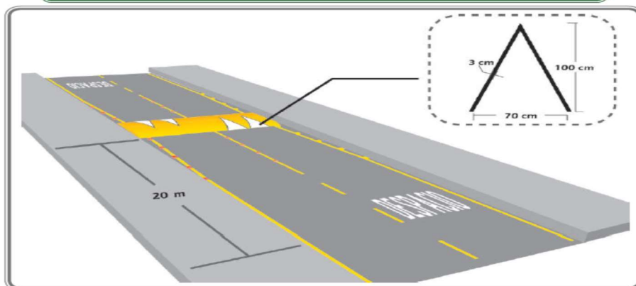
Figura 3-66 Reductor de Velocidad
