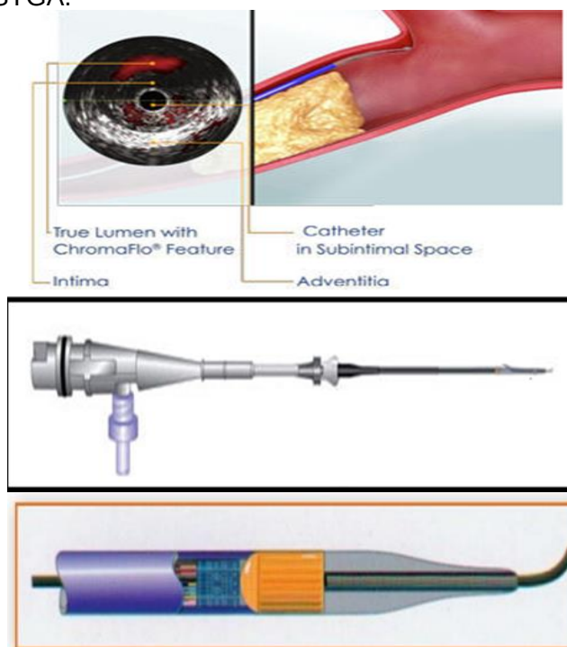
Imagen 2. Catéter Atlantis para Ultrasonido intravascular y ecografía intravascular. Tomado de: http://www.ecuasurgical.com/index.php/productos/por-marca/boston-scientific/atlantis%E2%84%A2-sr-pro-cat%C3%A9ter-de-ultrasonido-intravascular-de-un-solo-uso.html
