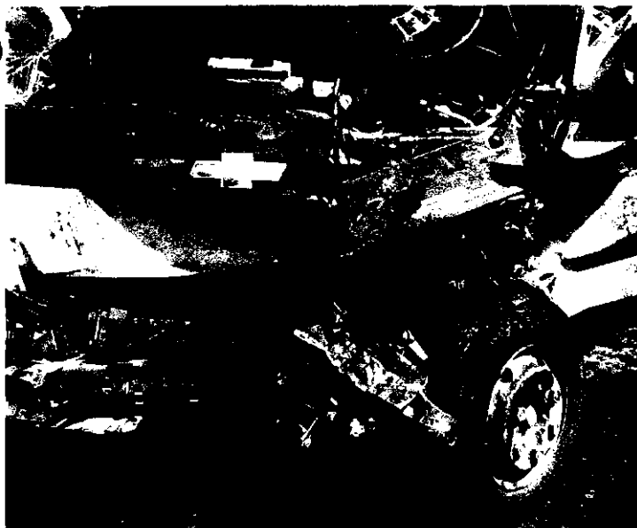
GRAFICA Nro. 02 y 03: Observamos su chasis torcido, cabina parte frontal totalmente destruida, su puerta lado izquierdo doblada y techo de cabina doblado.
