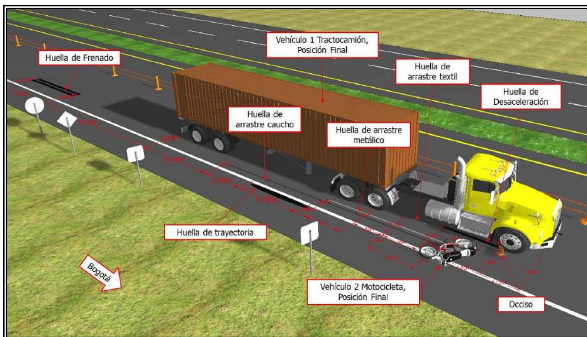
Imagen 2.18 Plano de la escena
