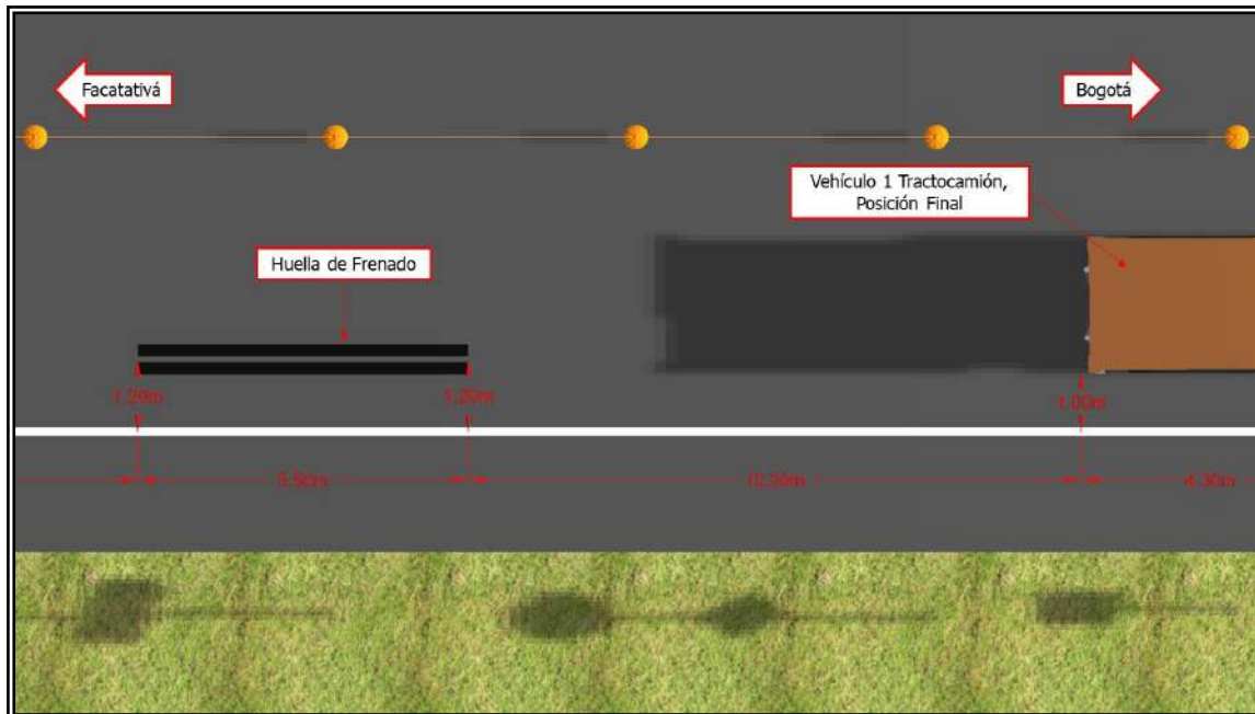
Imagen 2.13 Plano de la escena
