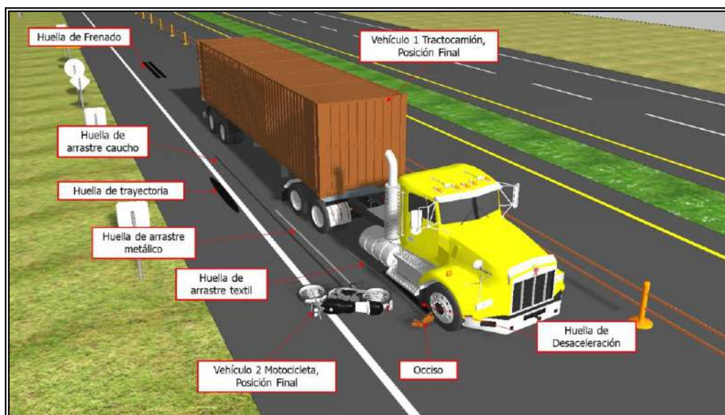
Imagen 4.11 Mecánica de Colisión
