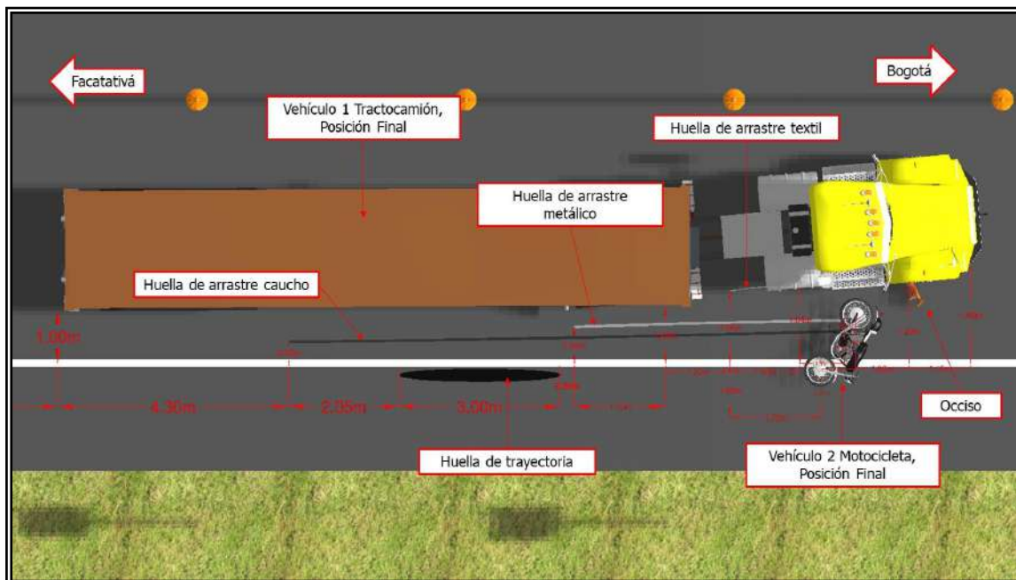
Imagen 2.14 Plano de la escena
