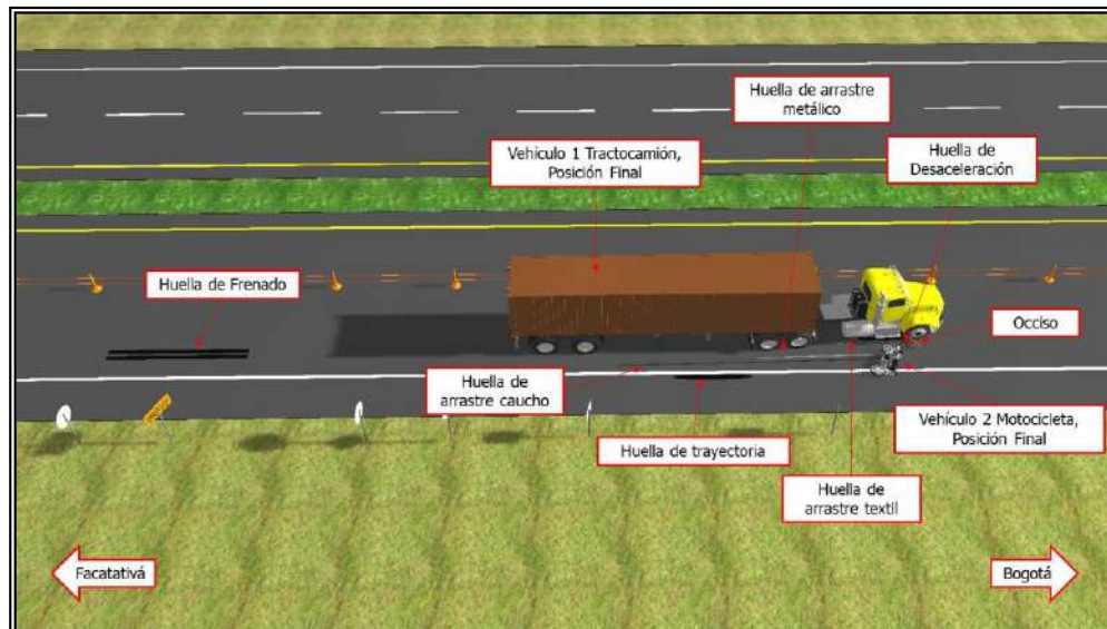
Imagen 4.10 Mecánica de Colisión
