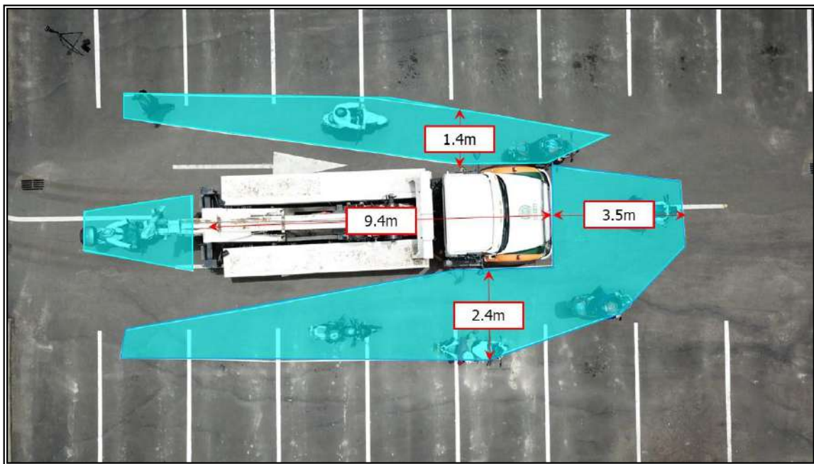
Imagen 4.15 Puntos ciegos Camión
