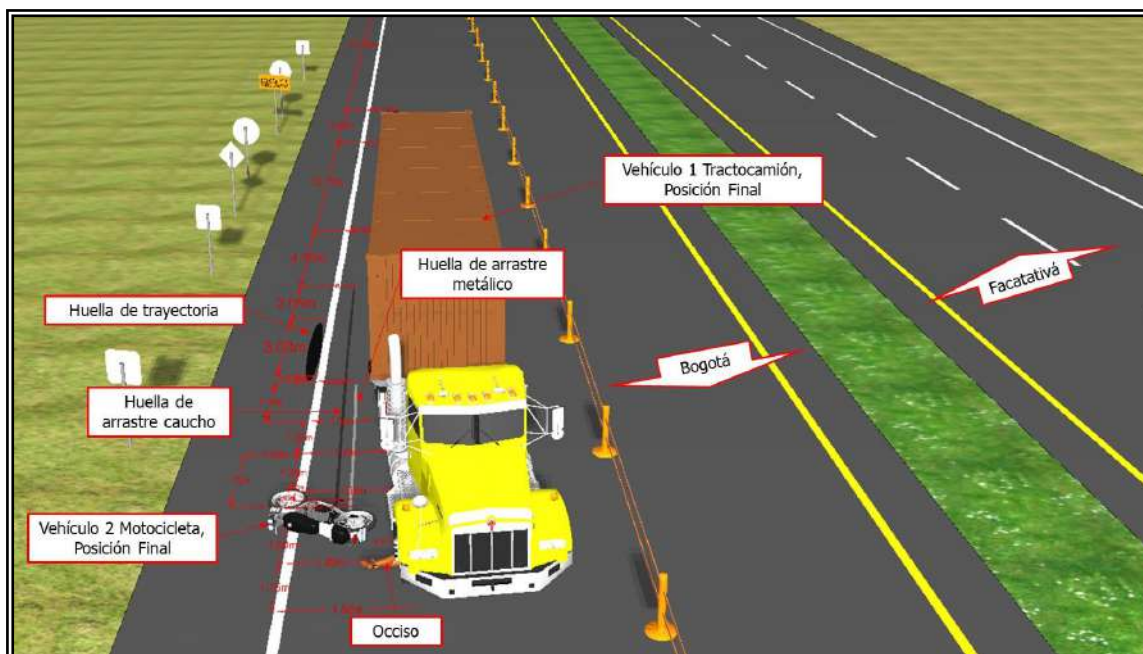
Imagen 2.17 Plano de la escena
