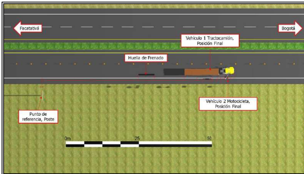
Imagen 2.11 Plano panorámico de la escena
