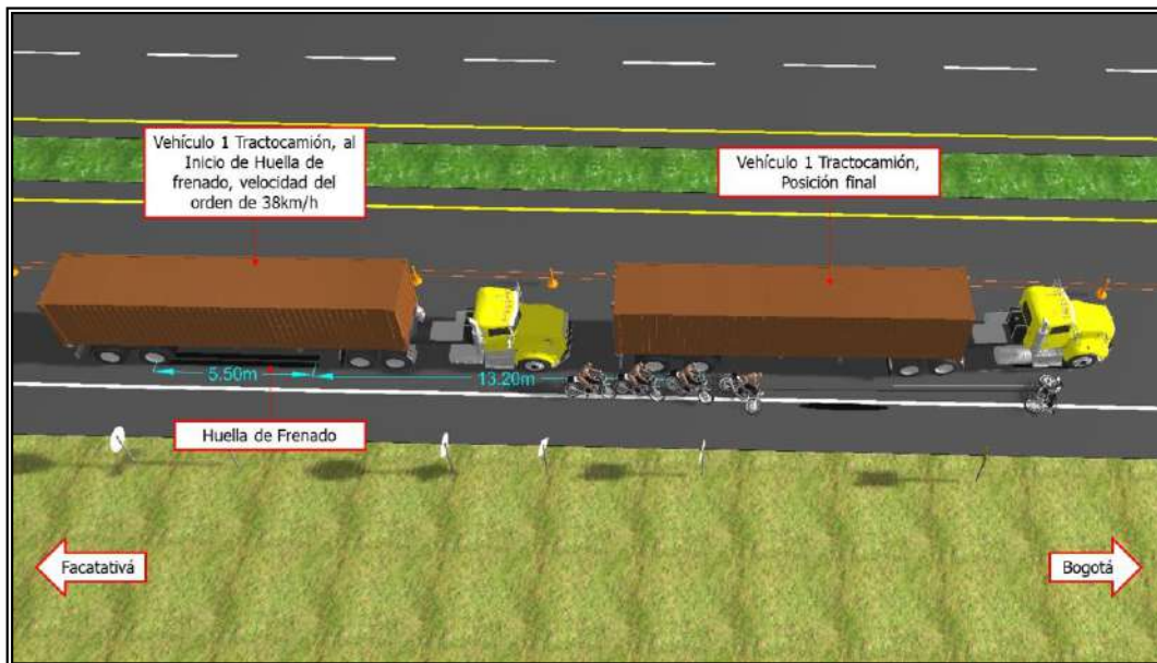
Imagen 4.12 Velocidad del vehículo 1
