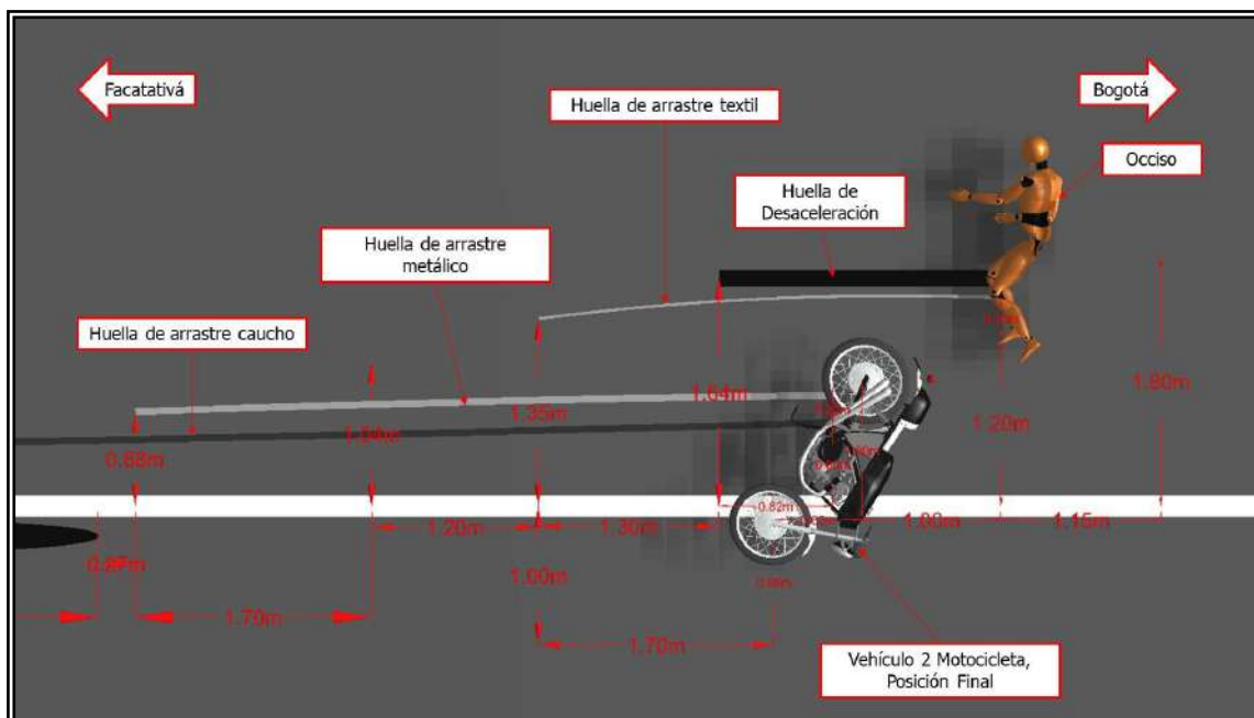
Imagen 2.15 Plano de la escena
