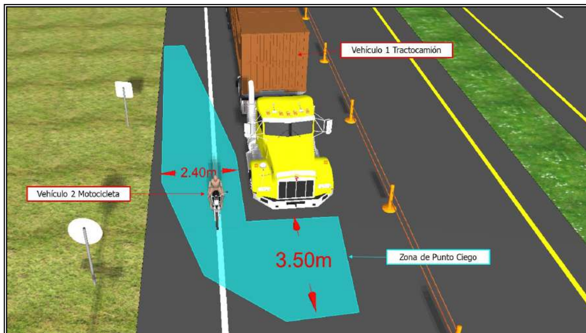
Imagen 4.17 Puntos ciegos Camión
