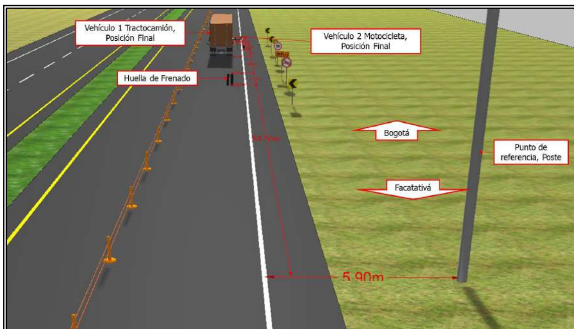
Imagen 2.16 Plano de la escena
