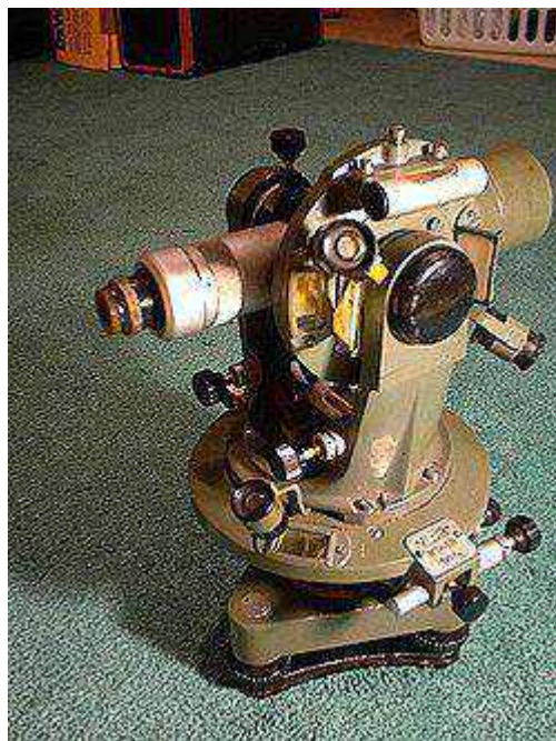
Teodolito soviético (URSS, 1958).
