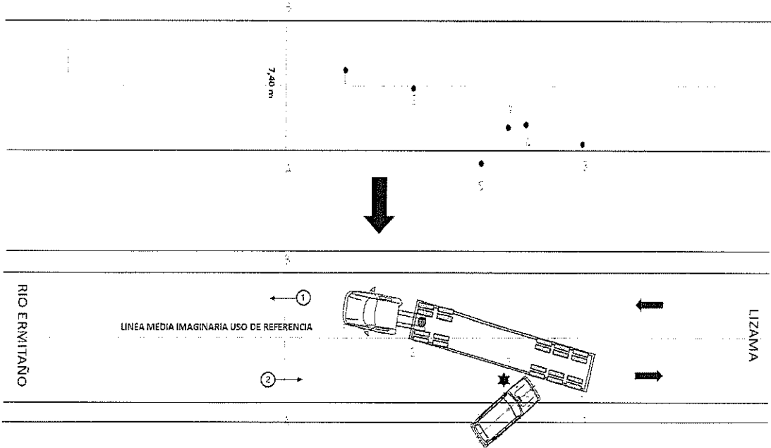
Imagen 6. Reconstruccion a escala del croquis, segun medidas reportadas en el mismo.
