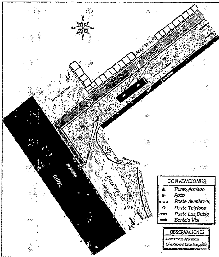
Imagen 13. Plano Topográfico 31447, en el cual, se detalla la acotación de los elementos materia de prueba (EMP) fijados por el personal investigativo del Centro Internacional Forense FCII que atendió el hecho (Bus de placa WGK 050 y cuerpo sin vida del señor CARLOS ALBERTO SORZA GARZON).
