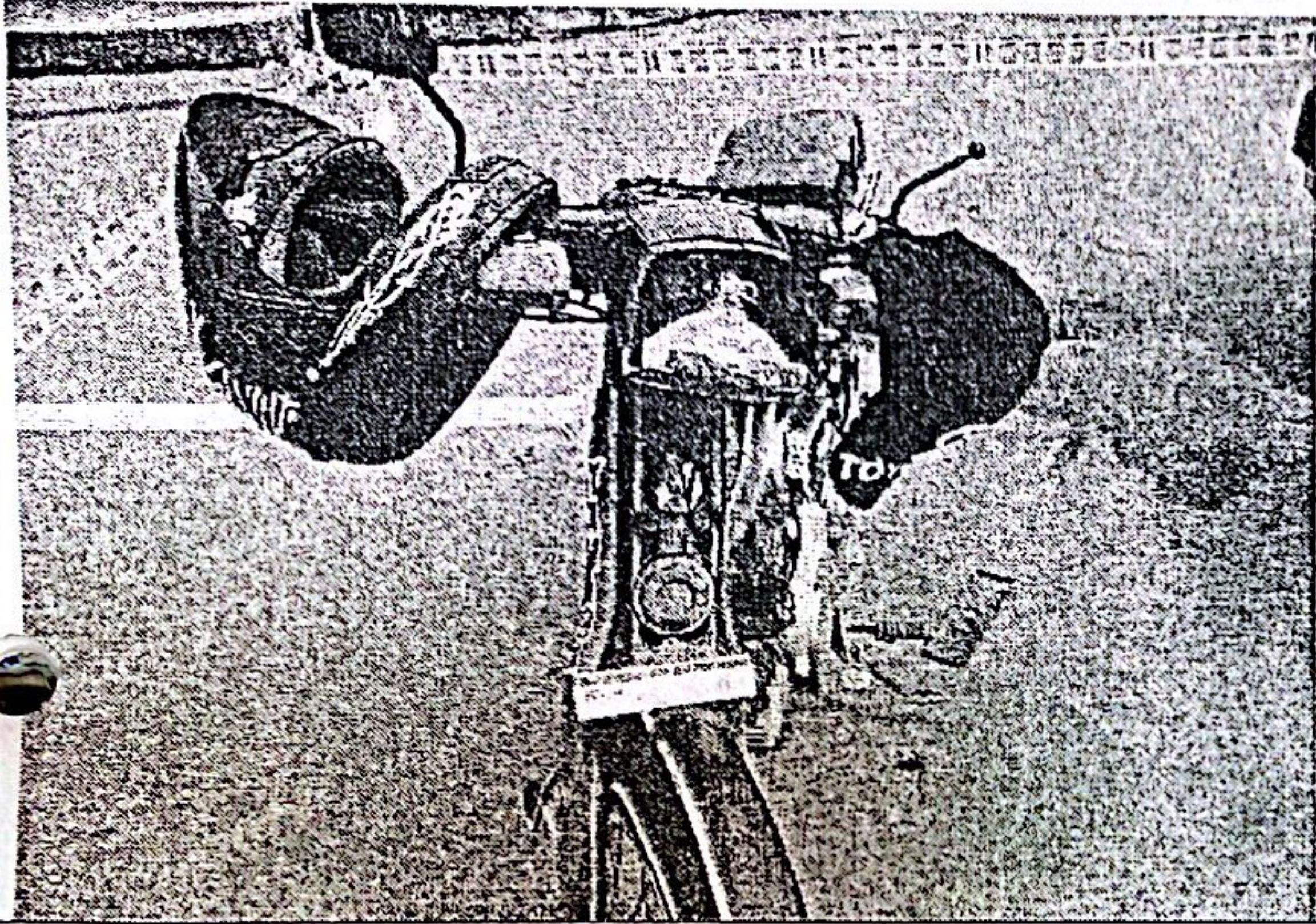
IMAGEN 5 TOMA P3240443 PRIMER PLANO: se aprecia la motocicleta implicada en el accidente, con daños generales causados por el impacto.
