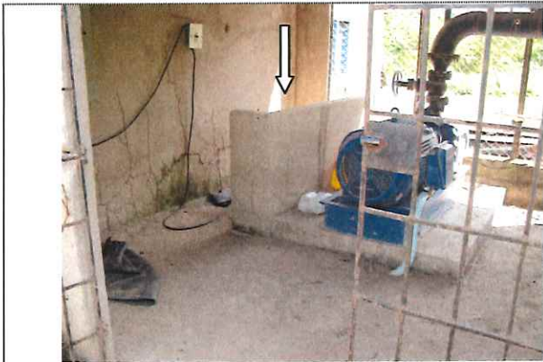
IMAGEN 5. Toma 105-7633, Plano General, se observa el motor trifásico tipo Turbina Industrial y una Turbina Electrica comercial (pequeña) y su respectiva conexión eléctrica.
