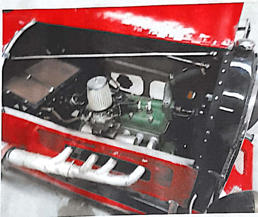
9.- Motor del vehículo lado derecho, radiador y tubo de escape.
