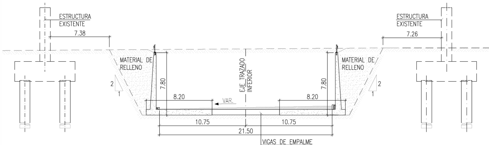
SECCIÓN TÍPICA PROPUESTA 1 – DEPRIMIDO ESCALA: 1/150 PLIEGO
