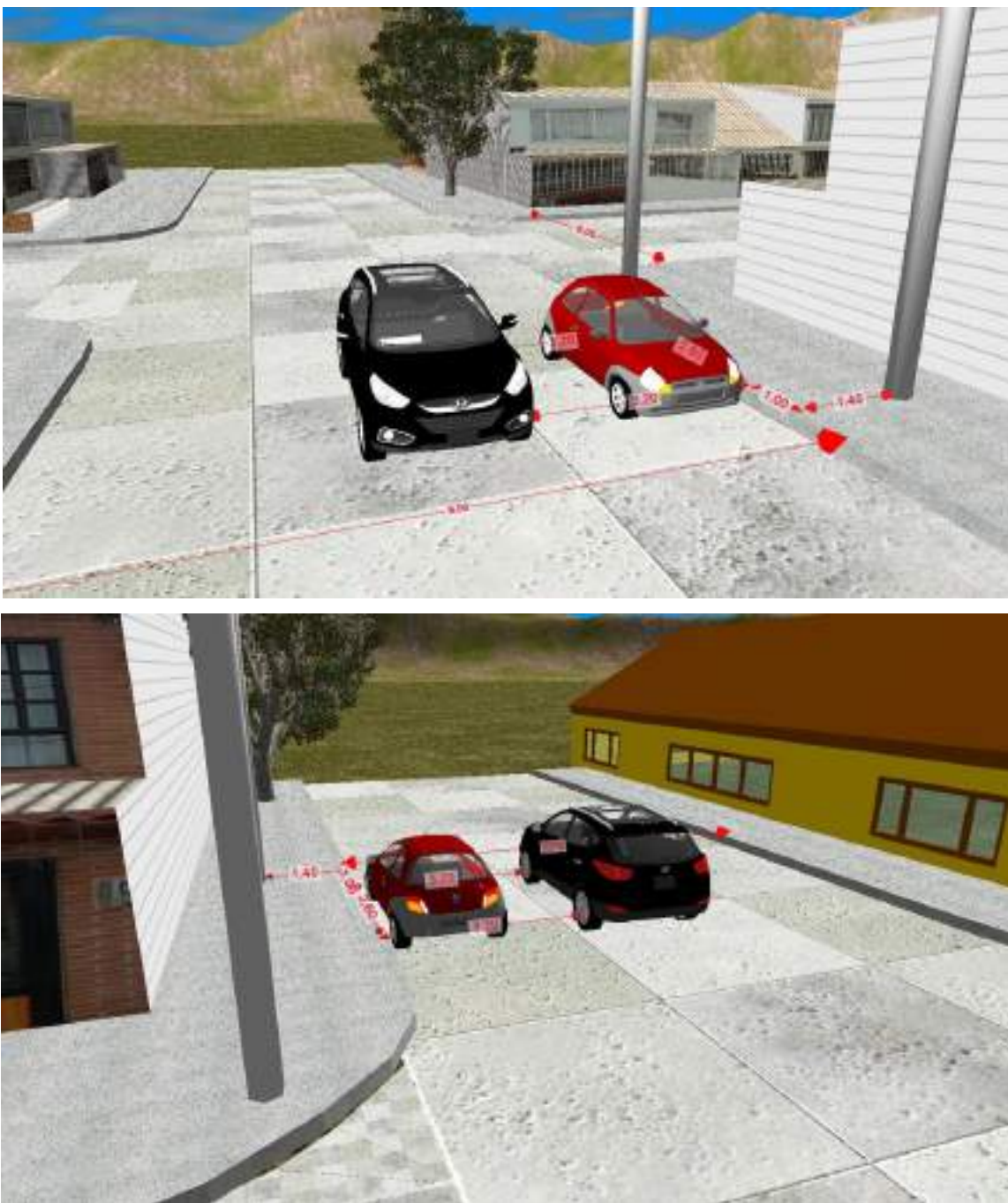
Imagen No. 12: En estas imágenes en 3D se observan las evidencias diagramadas en el croquis de la autoridad. Elaboración a escala en el software Trimble Forensics Reveal.
