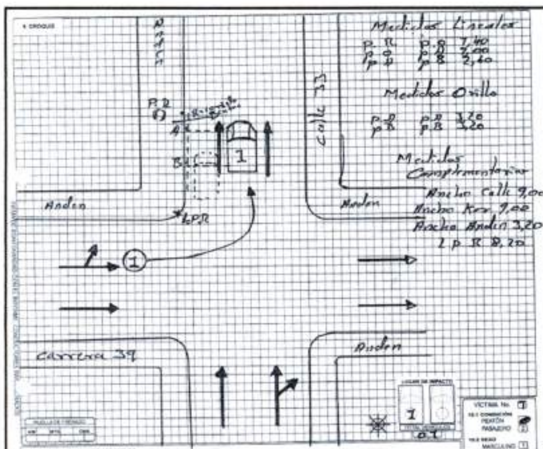
IMAGEN No. 8: En esta imagen se muestra el croquis del accidente realizado por la autoridad de tránsito.
