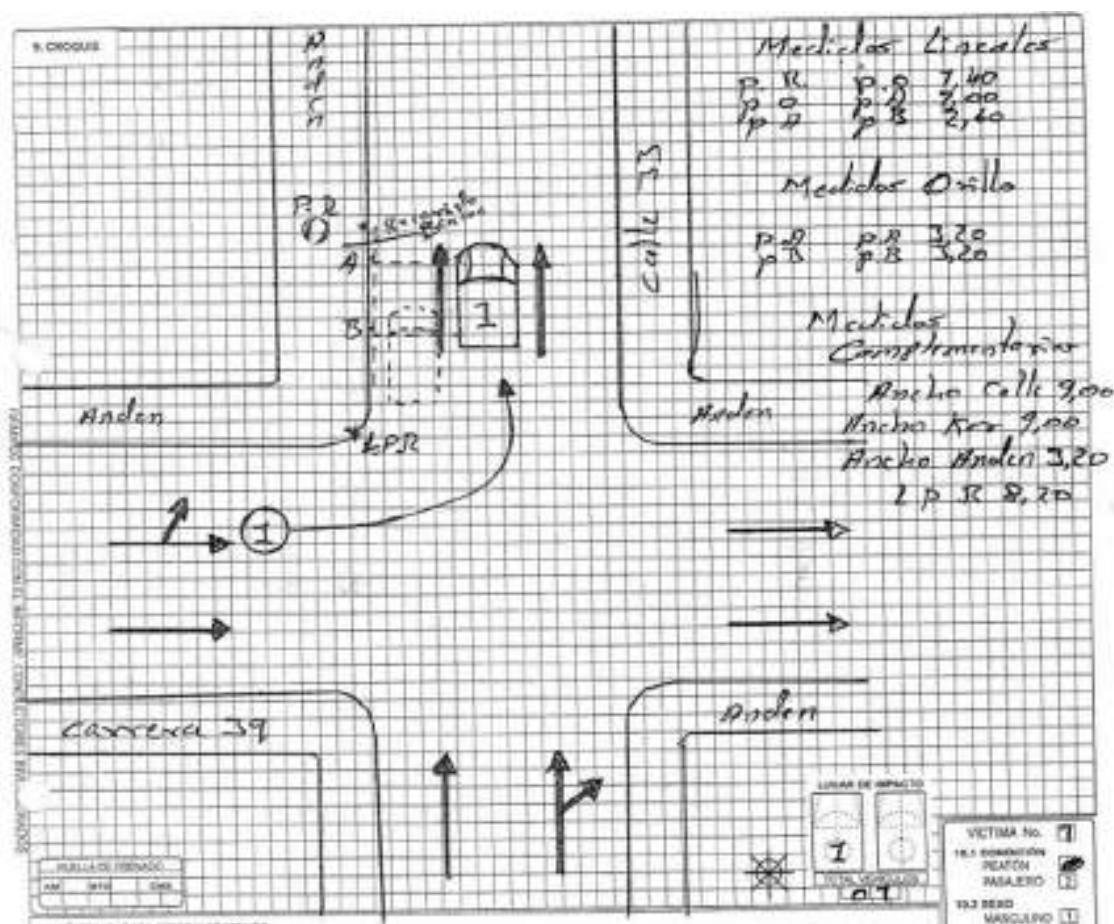
Imagen No. 10: En esta imagen se muestra el croquis del accidente realizado por la autoridad de tránsito.
